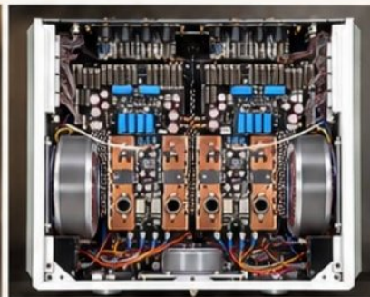
SOULNOTE A-3 VISTA INTERIOR
