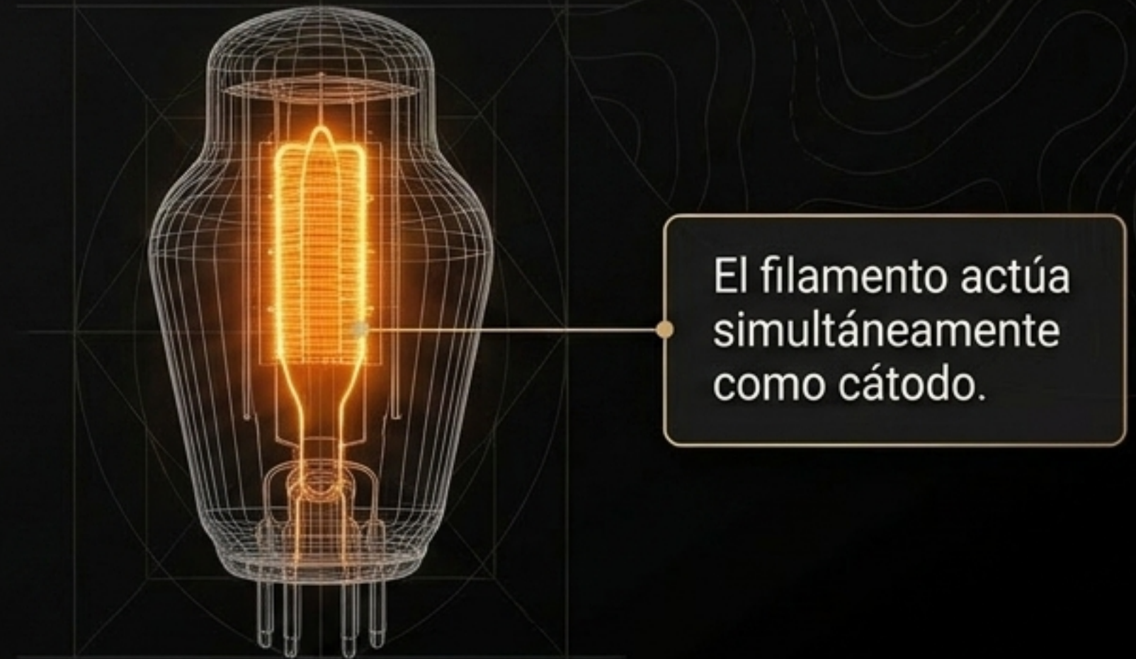
La 300B
