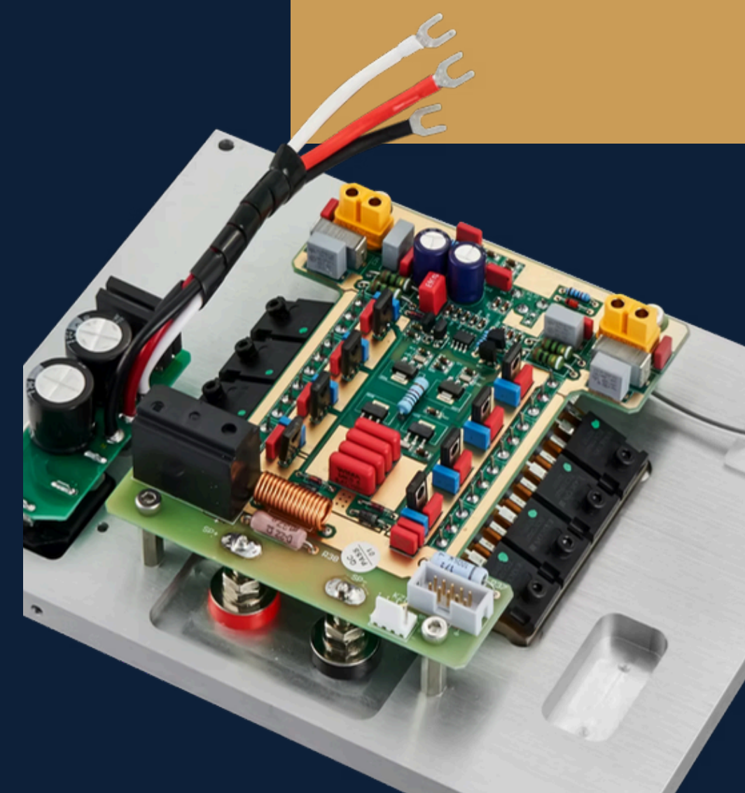
MOSFET EXICON
